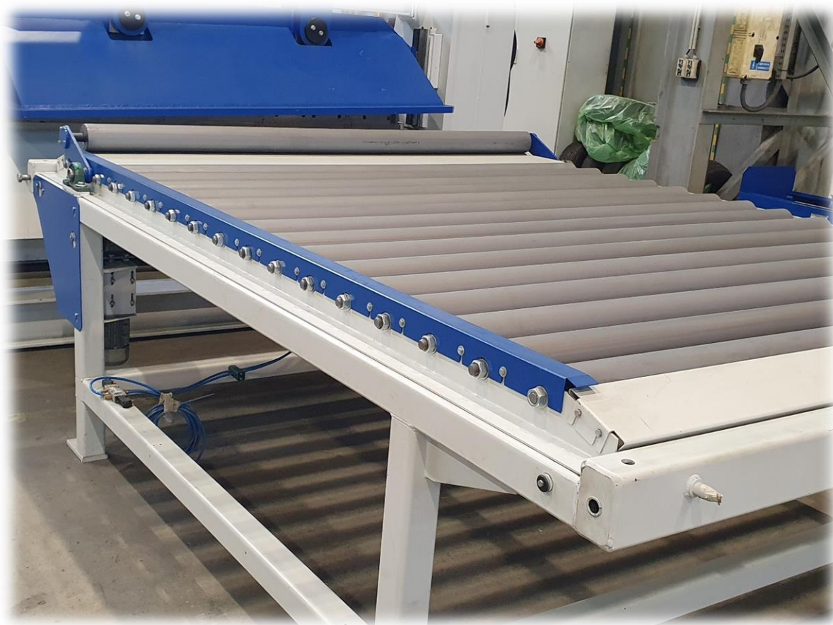
Rys. 5-7 – Transporter wylotowy segmentowy
