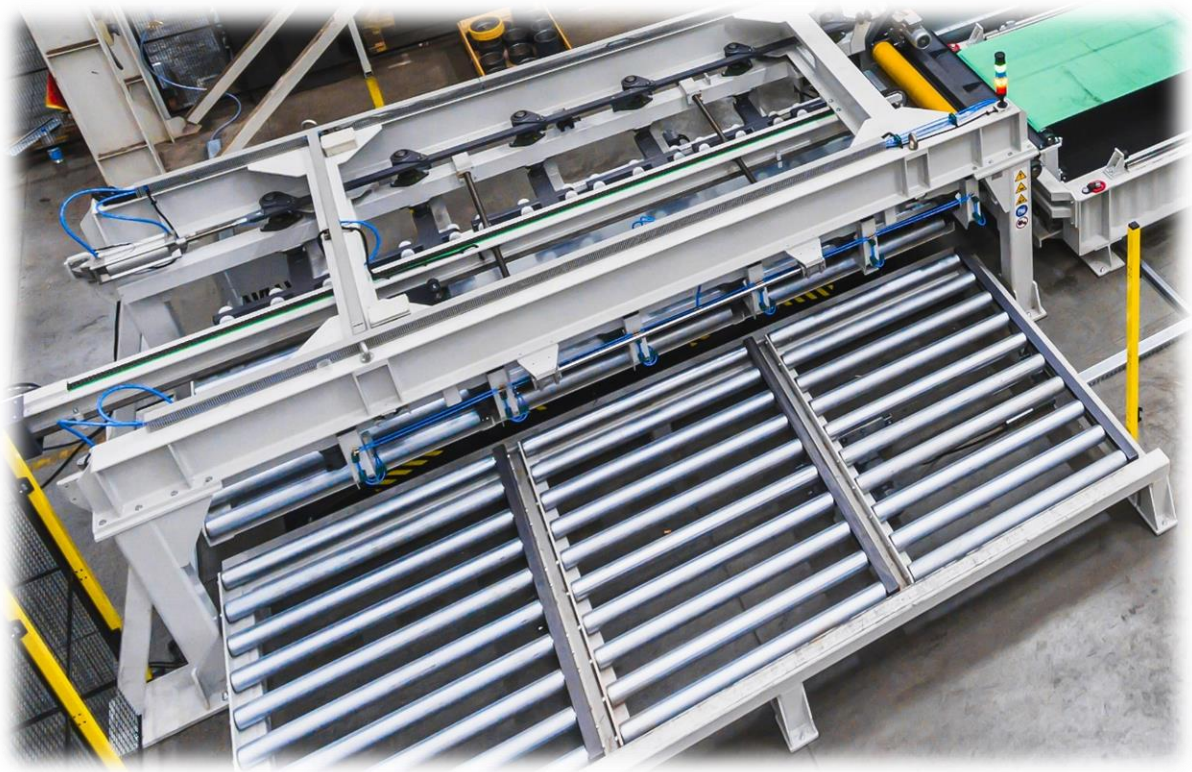
Rys. 5-8 – Moduł automatycznego układania arkuszy, przykład wykonania
