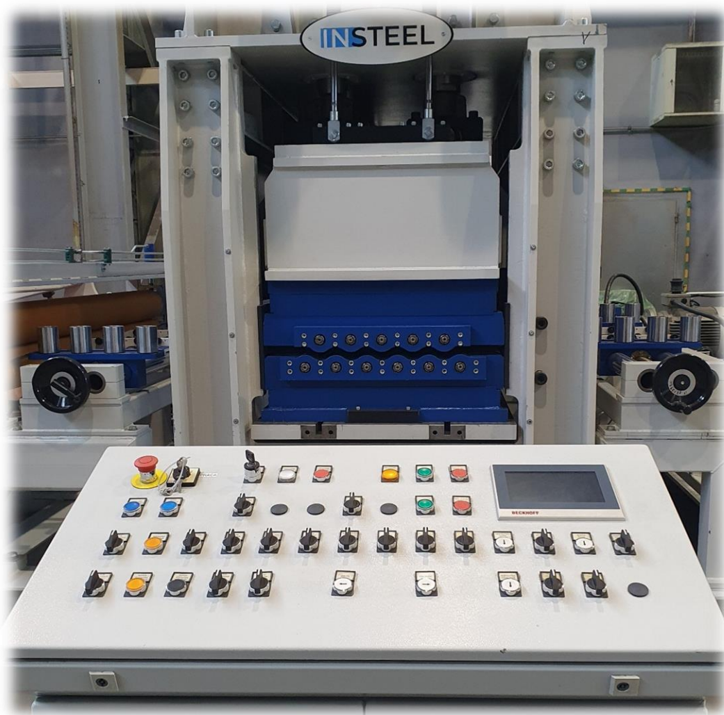
Rysunek 5-10 – Pulpit sterowniczy
